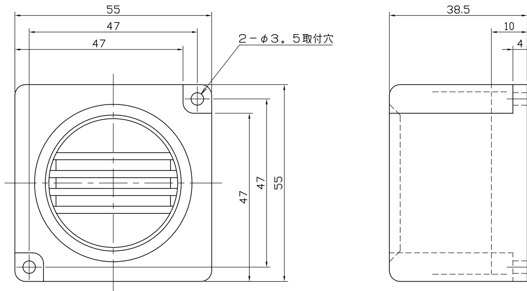
正面図
