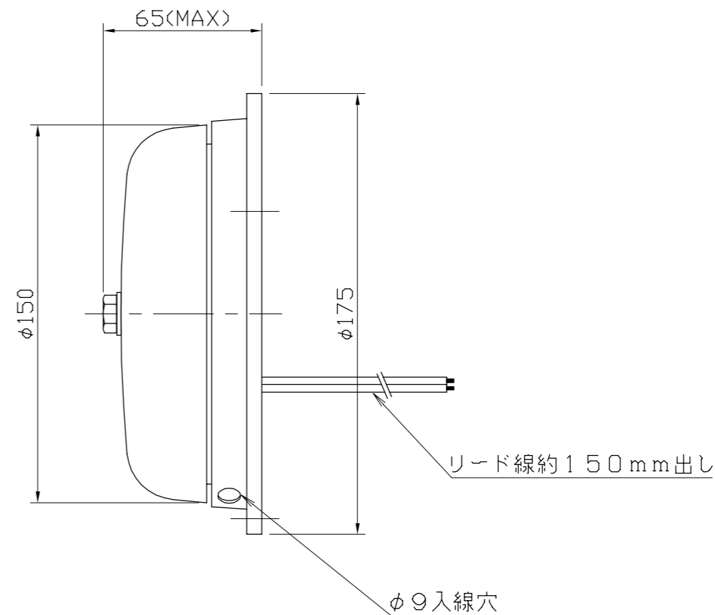
側面図
