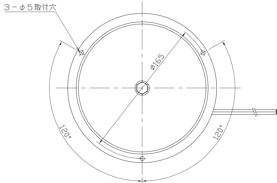
正面図
